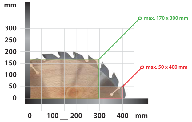
BL 170 Ø 600 mm
