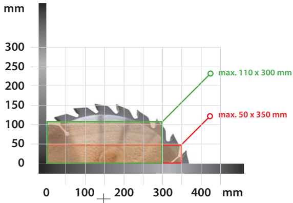
BL 225 Ø 700 mm
